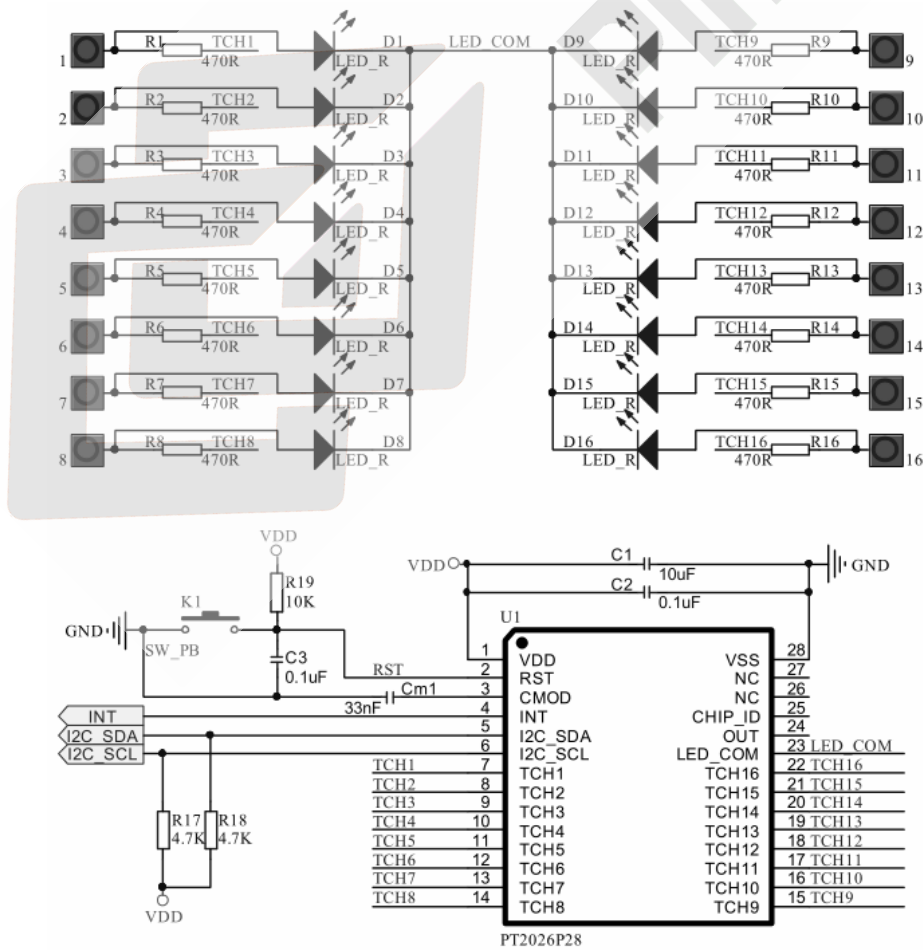
图 3 触摸复用 LED 驱动典型应用电路
