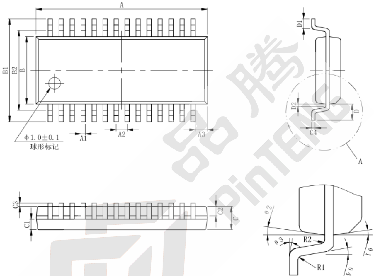
图 4 SSOP28 封装图
