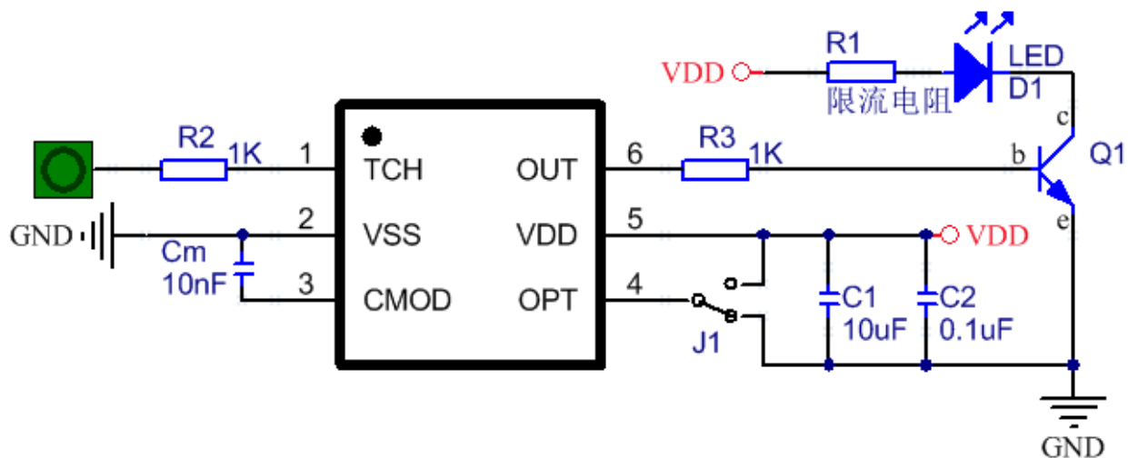
图 1 标准应用电路
