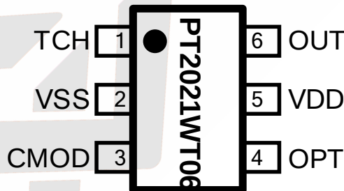
图 1 管脚示意
