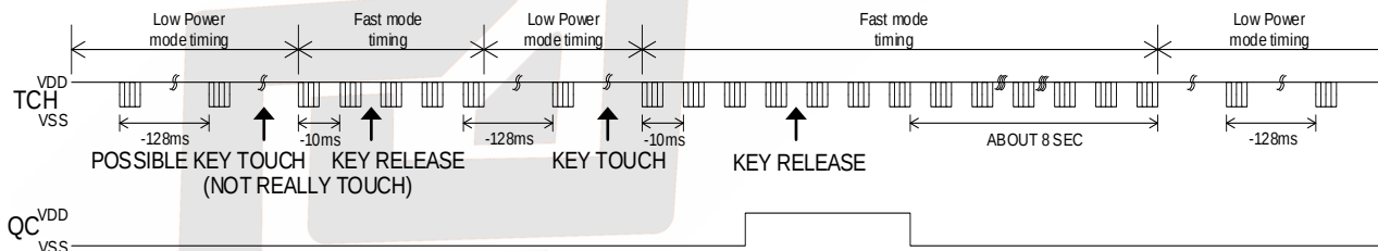
图 3 时序图
