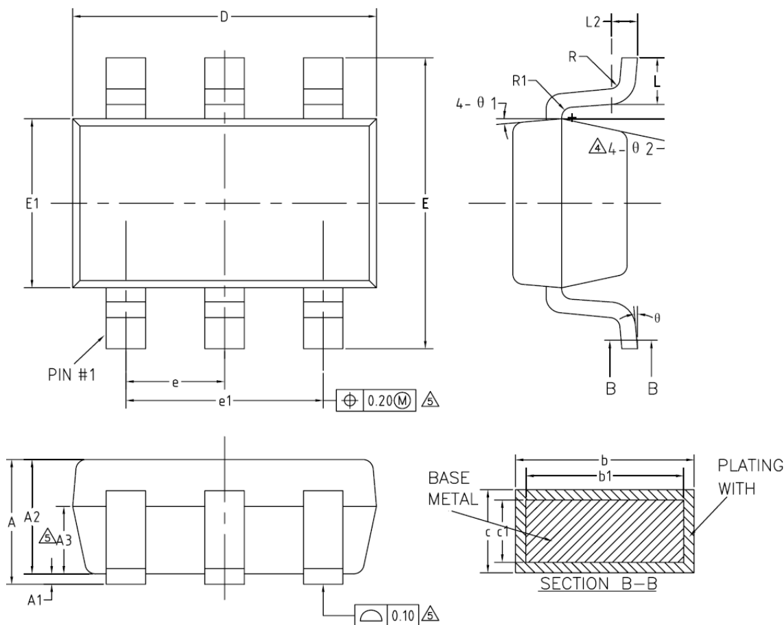
图 5 SOT23-6 封装图
