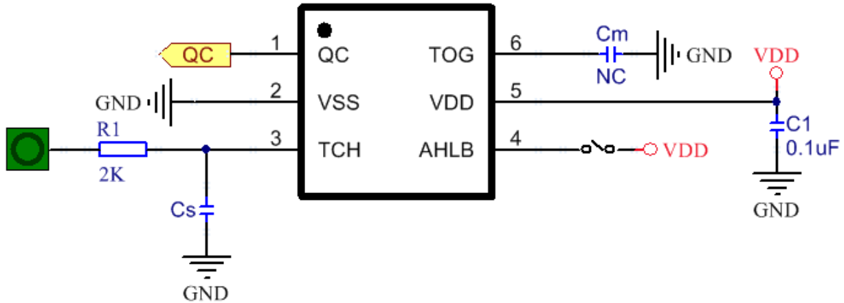
图 4 电路示意图
