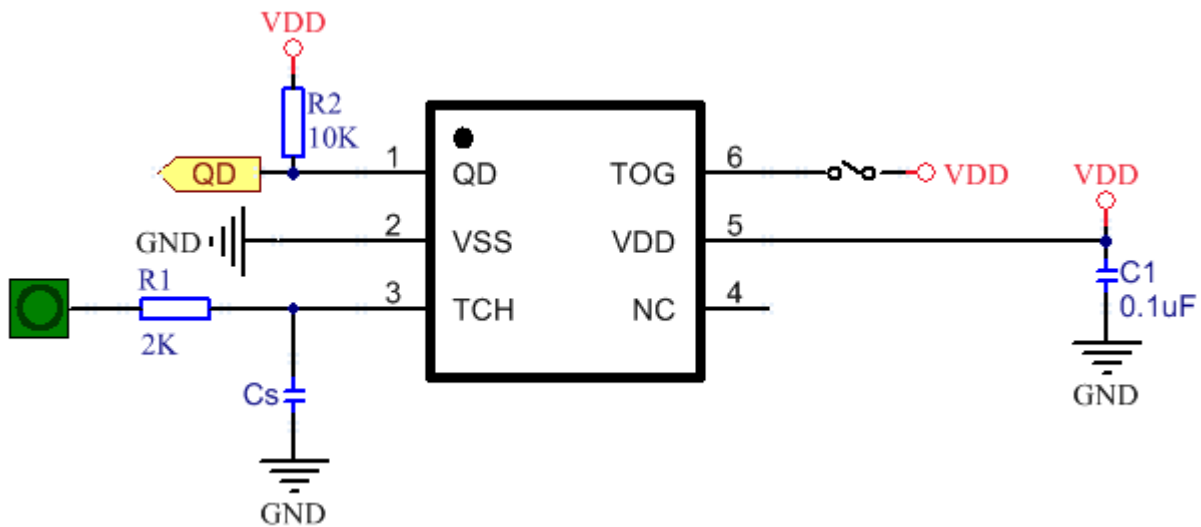
图 4 电路示意图
