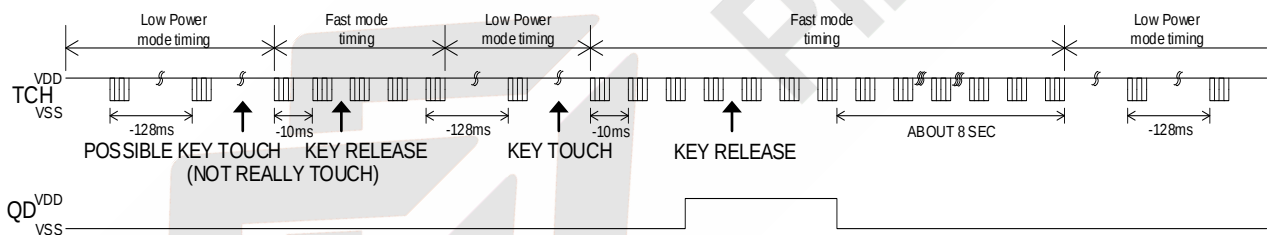
图 3 时序图
