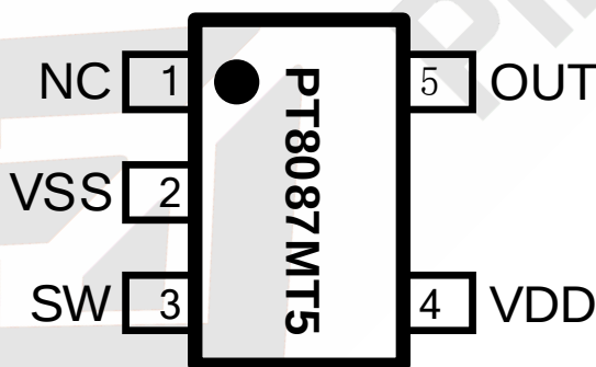
图 1 管脚示意图
