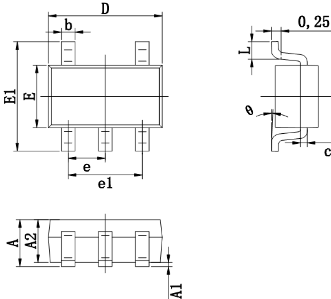
图 7 SOT23-5 封装图
