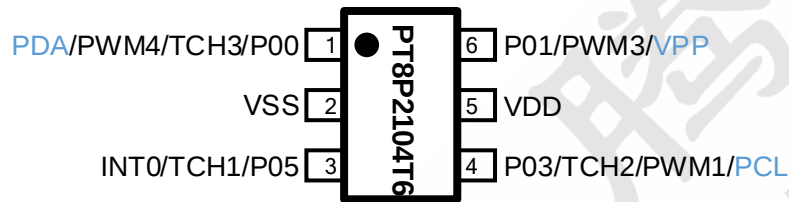
图 1 封装示意图
