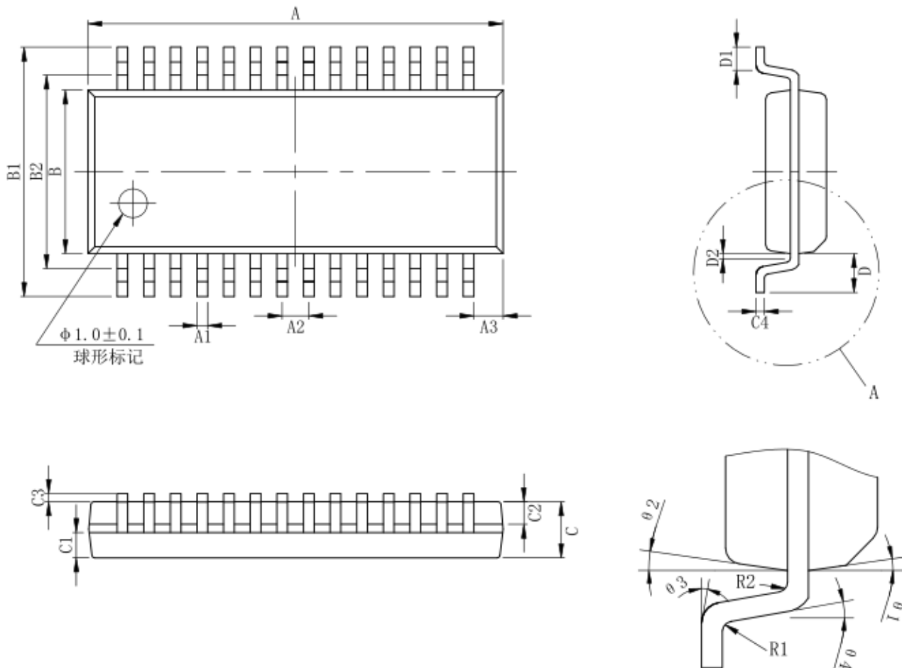
图 4 SSOP28 封装图
