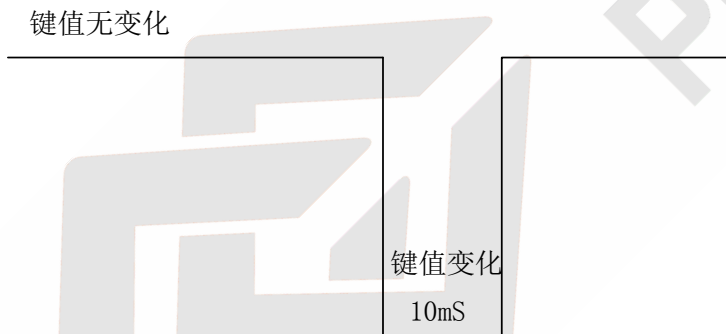
图 2 INT 端口信号示意图
