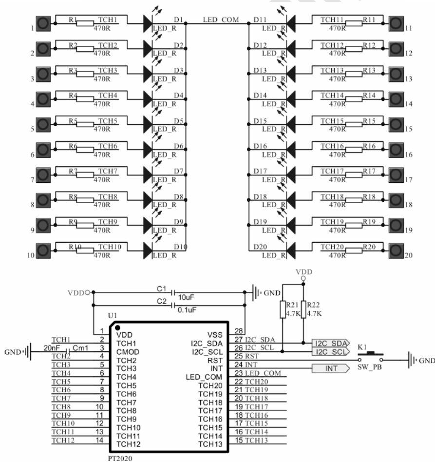
图 4 触摸复用 LED 驱动典型应用电路
