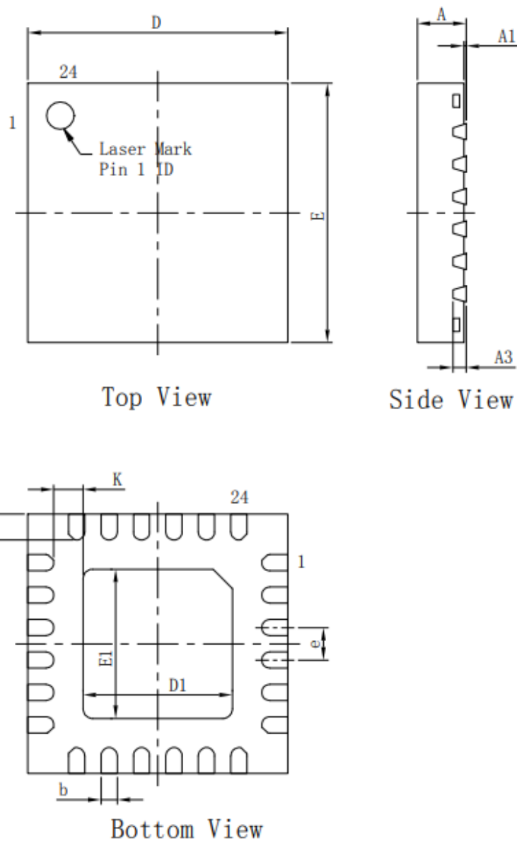
图 6 QFN24 封装图
