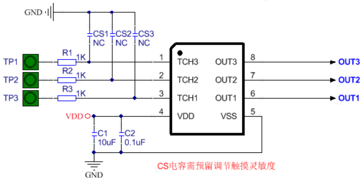
图 2 典型应用电路
