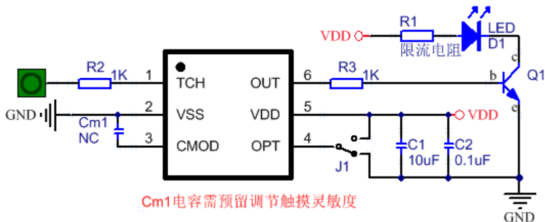
图 2 标准应用电路
