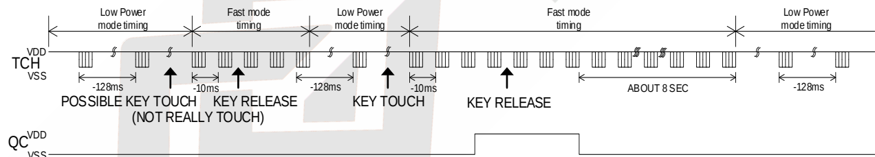
图 4 时序图
