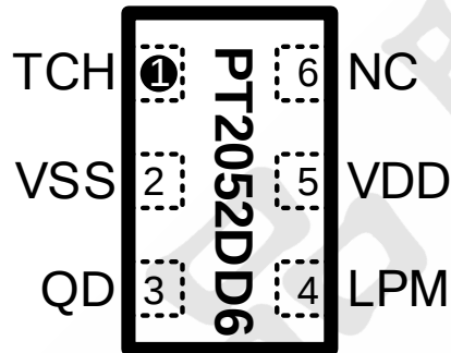
图 3 DFN2x2-6L 管脚示意图
