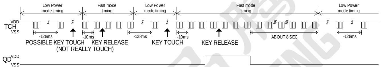
图 6 时序图
