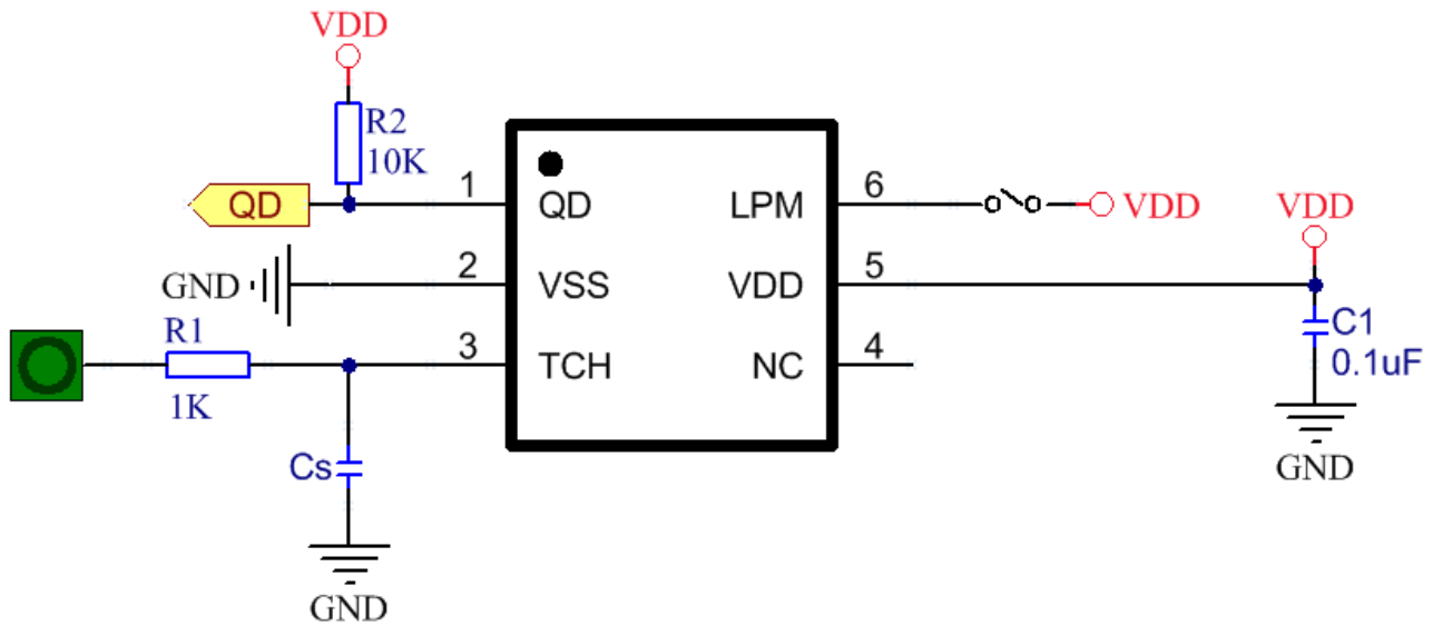
图 7 电路示意图
