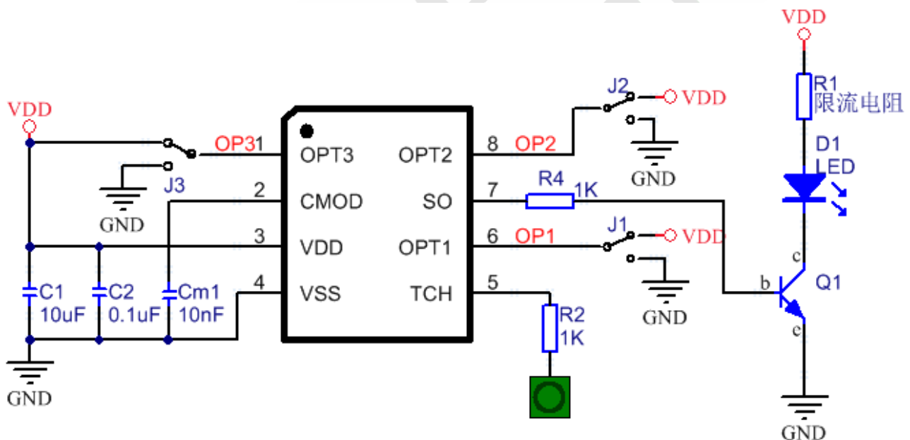
图 2 标准应用电路
