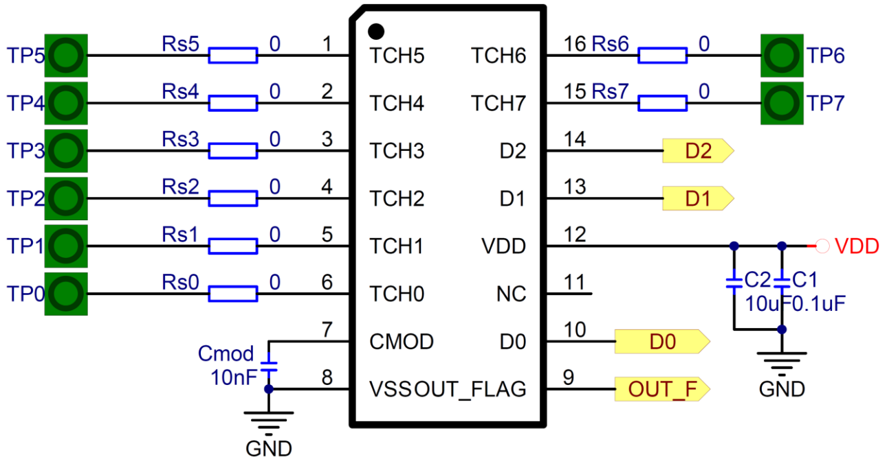
图 2 典型应用电路
