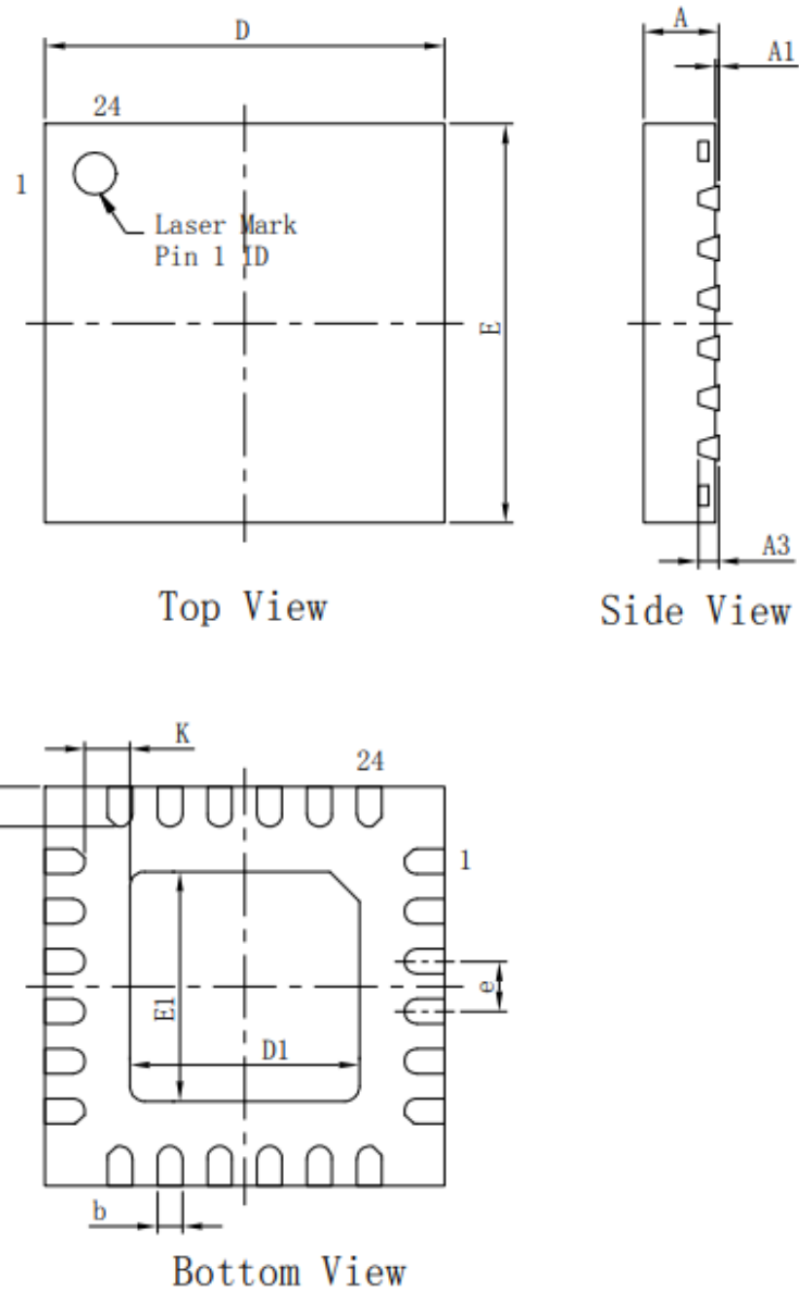
图 6 QFN24 封装图
