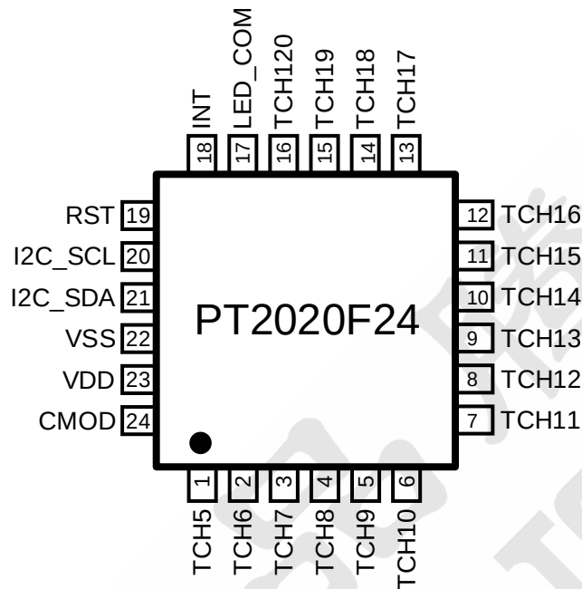
图 1 管脚示意
