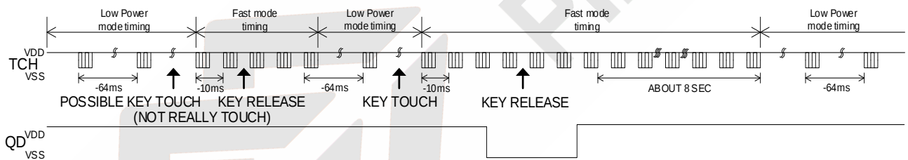
图 4 时序图
