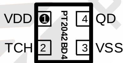
图 4 DFN1x1-4L 封装管脚示意图
