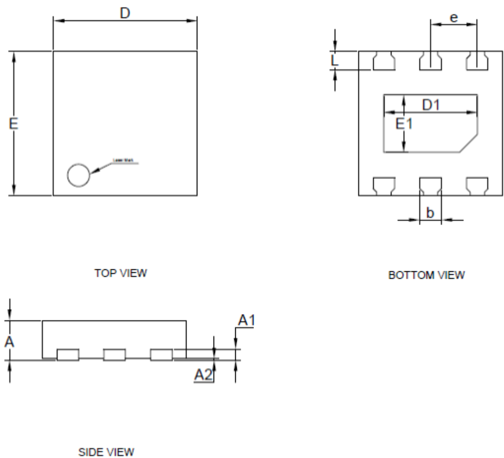
图 7 DFN2x2-6L 封装图
