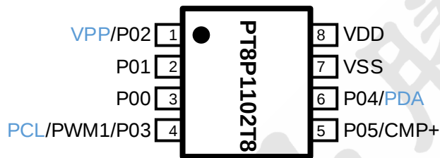
图 2 SOT23-8 封装示意图
