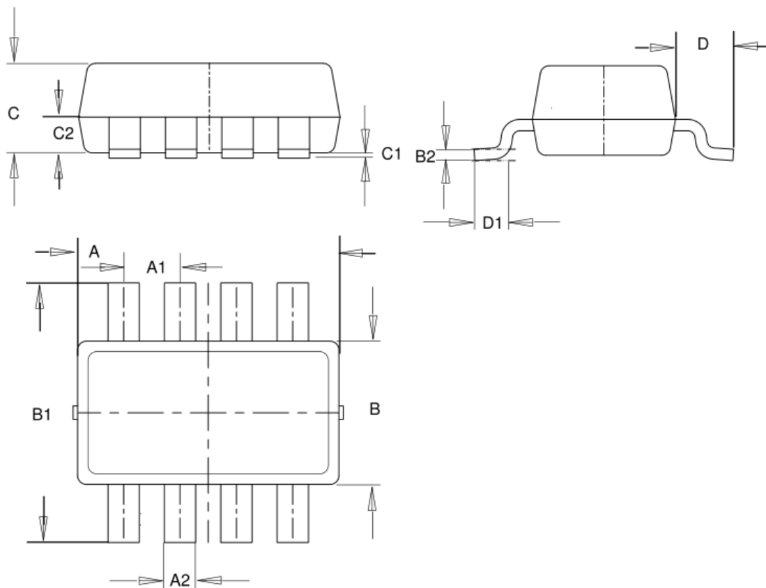
图 9 SOP8 封装图
