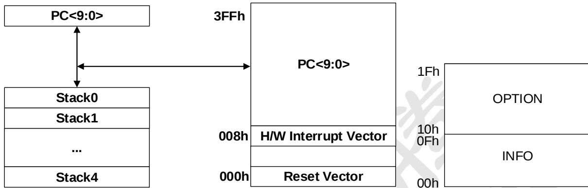
图 5 程序存储器 ROM 及 INFO 区
