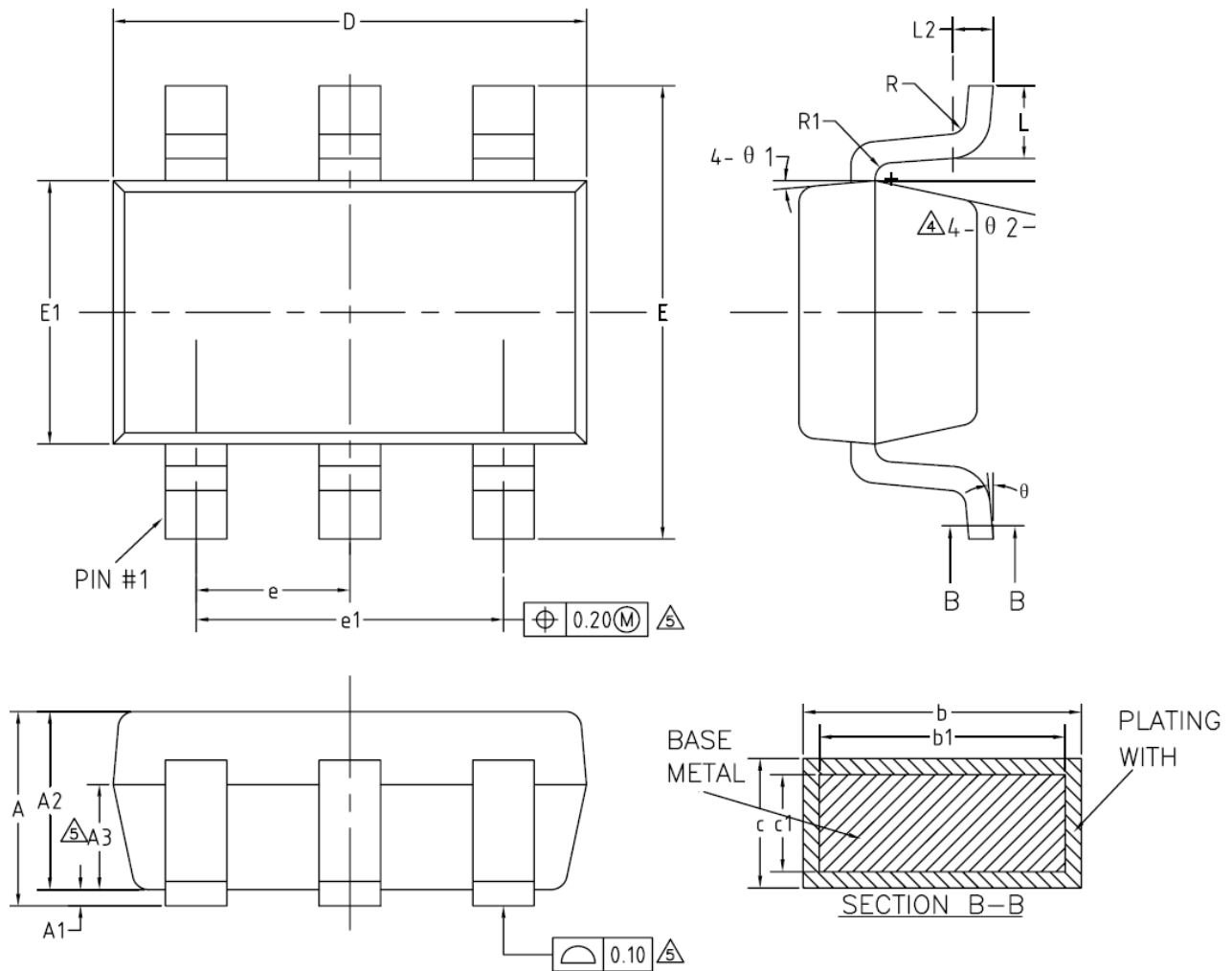
图 8 SOT23-6 封装图
