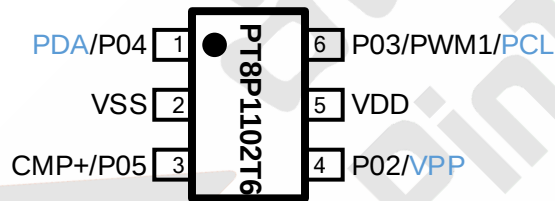
图 3 SOT23-6 封装示意图
