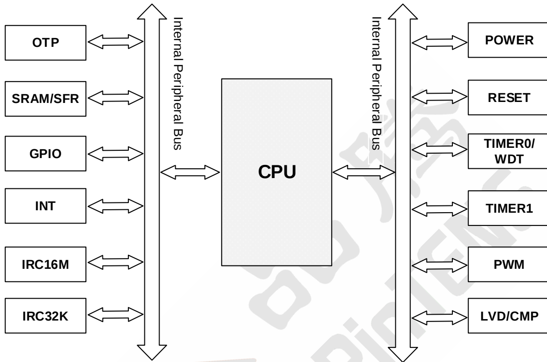
图 4 系统框图
