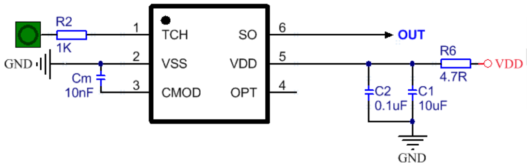
图 2 标准应用电路
