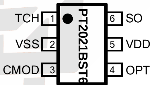
图 1 SOT23-6 封装示意图
