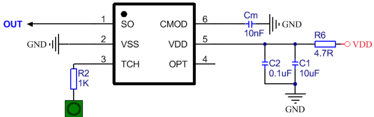
图 2 标准应用电路
