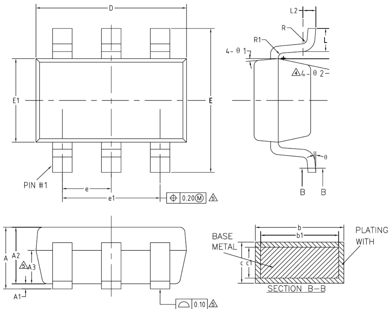
图 2 SOT23-6 封装
