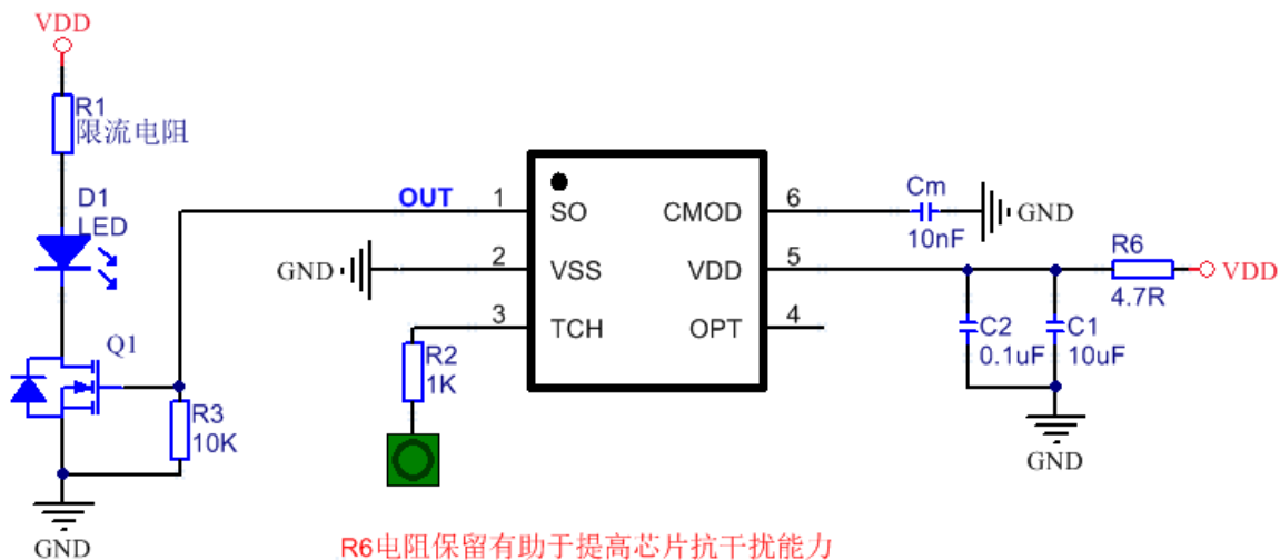
图 1 标准应用电路
