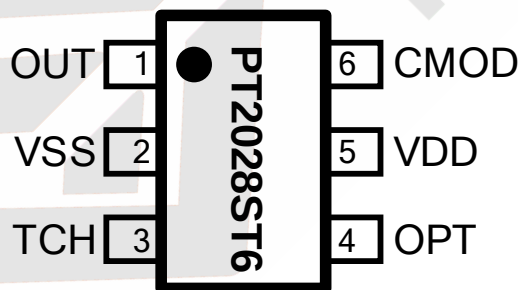
图 1 SOT23-6 封装示意图
