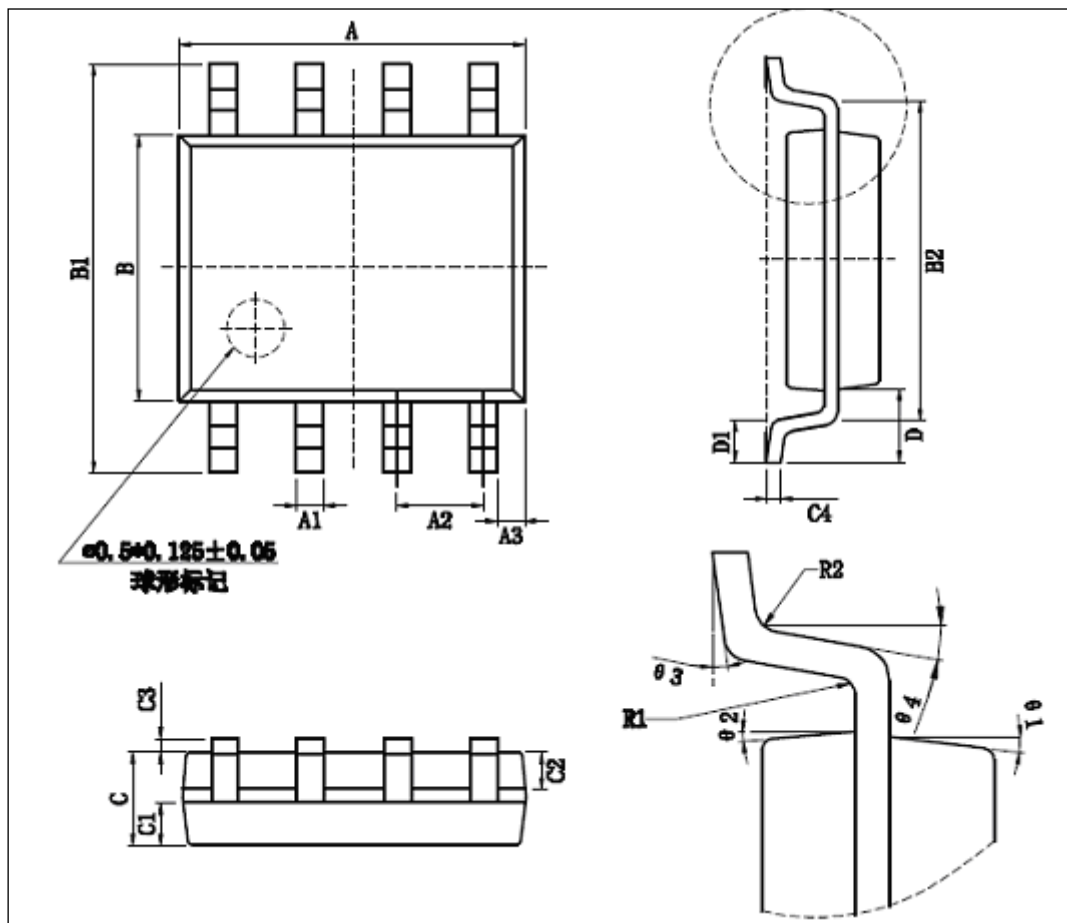
图 5 SOP8 封装图
