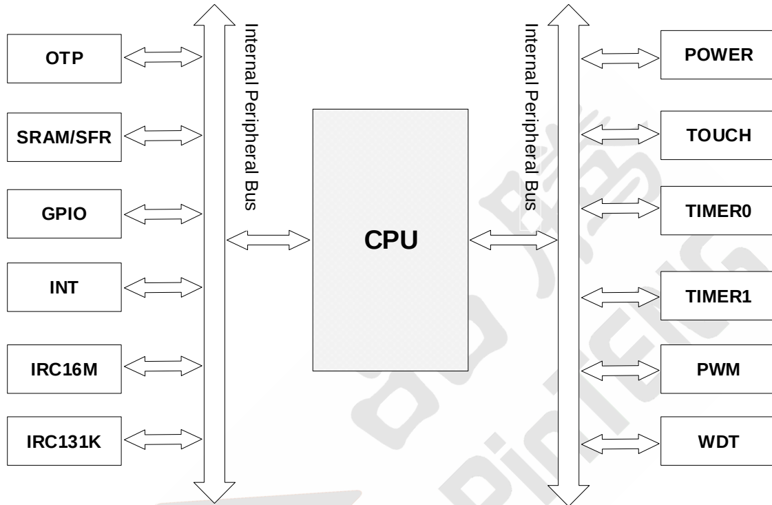
图 3 系统框图
