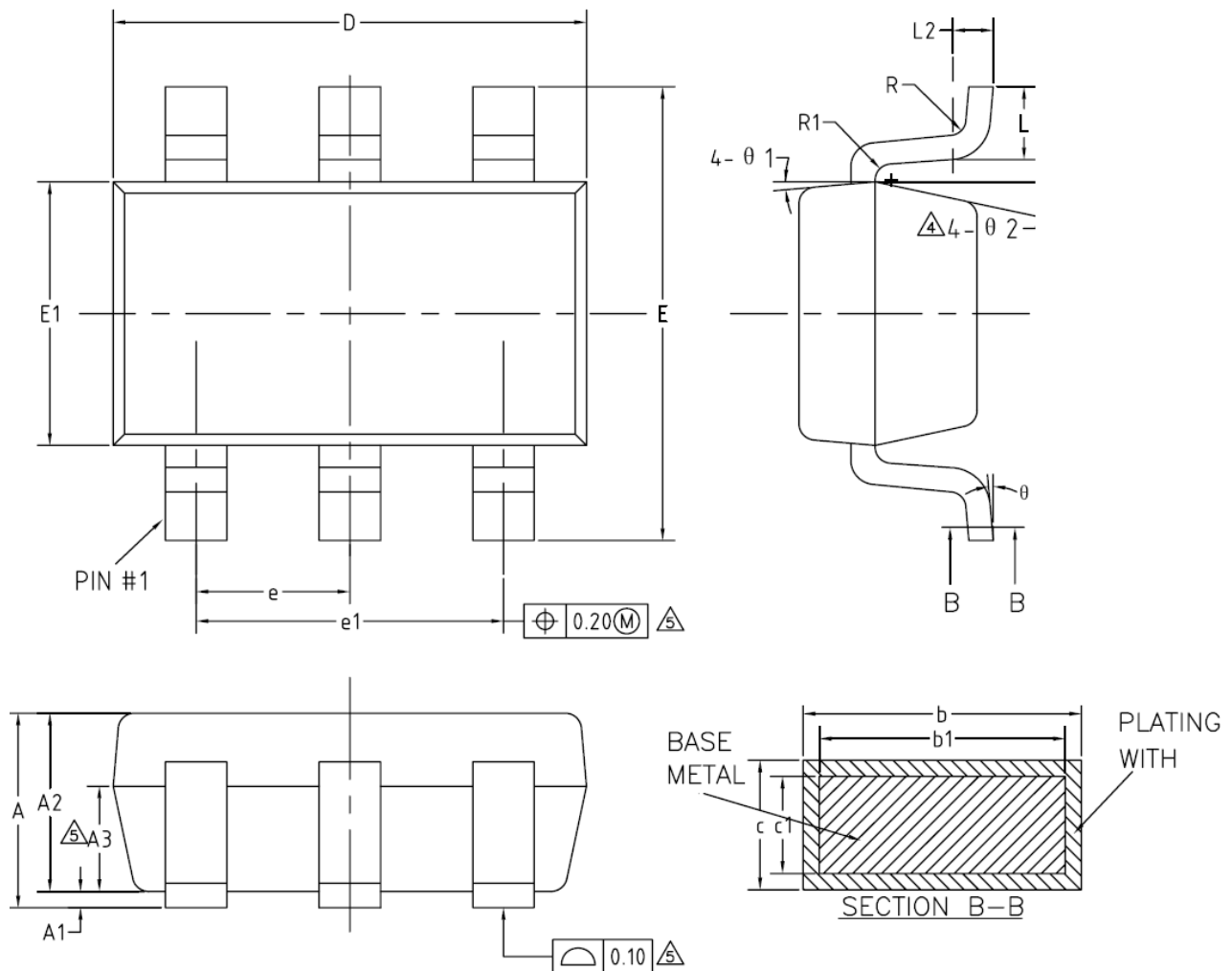
图 7 SOT23-6 封装图
